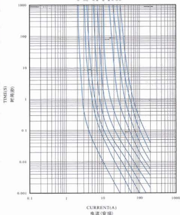
I-T CHARACTERISTICS CURVE 电流-时间曲线图
