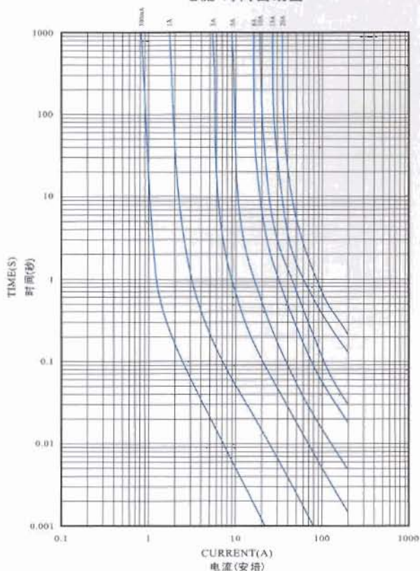
I-T CHARACTERISTICS CURVE 电流-时间曲线图
