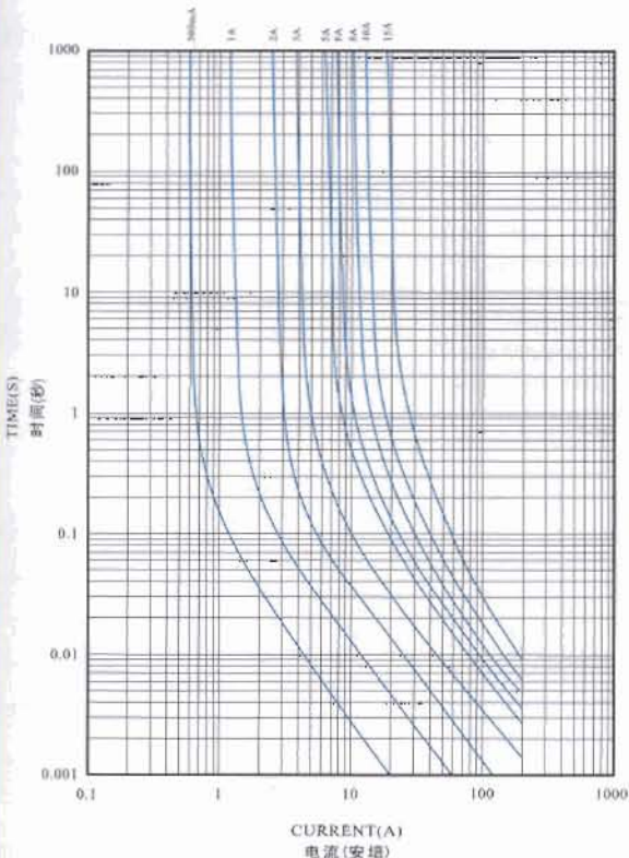
I-T CHARACTERISTICS CURVE 电流-时间曲线图
