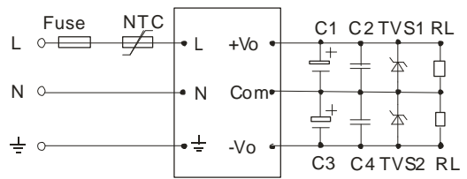
LH**-10A**(Dual output)
