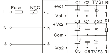
LH**-10C**(Triple Output)
